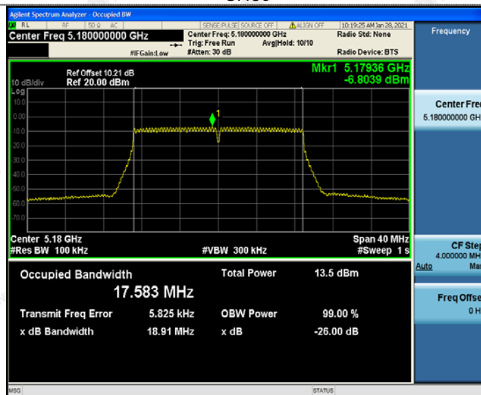
802.11 n HT 20
