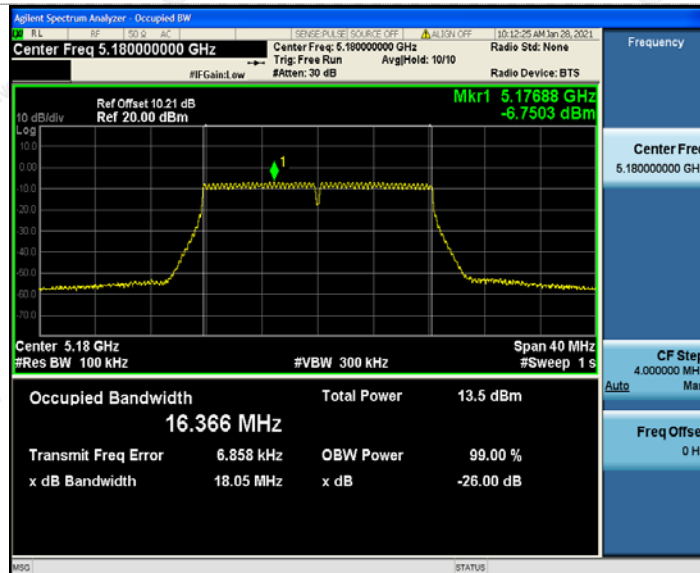
802.11 n HT 20
