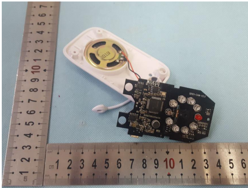
EUT Photo 6
