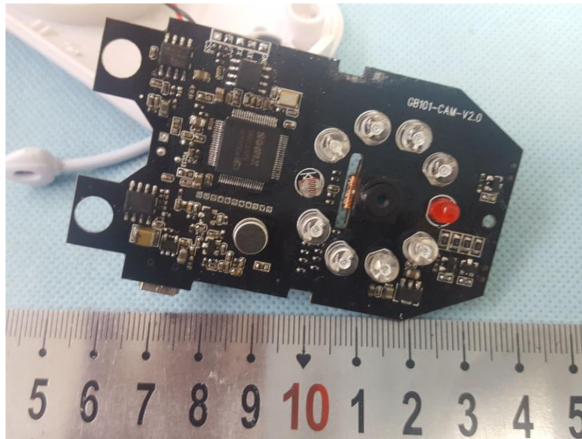
EUT Photo 7
