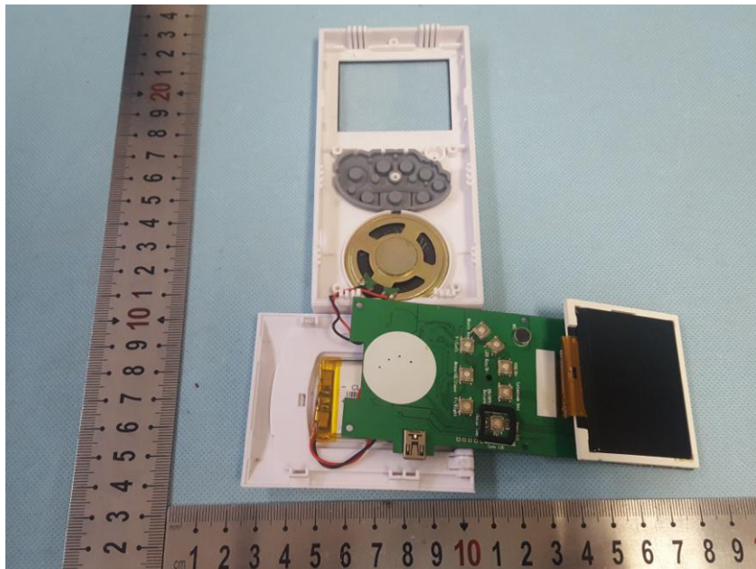
EUT Photo 4
