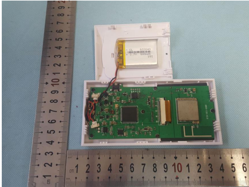
EUT Photo 3
