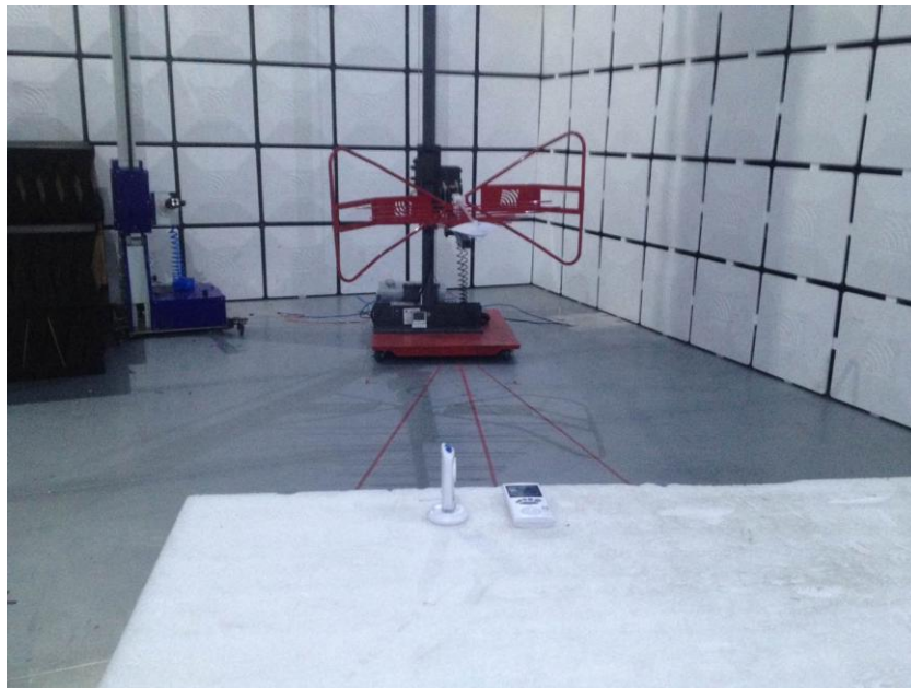
EUT Photo 8
