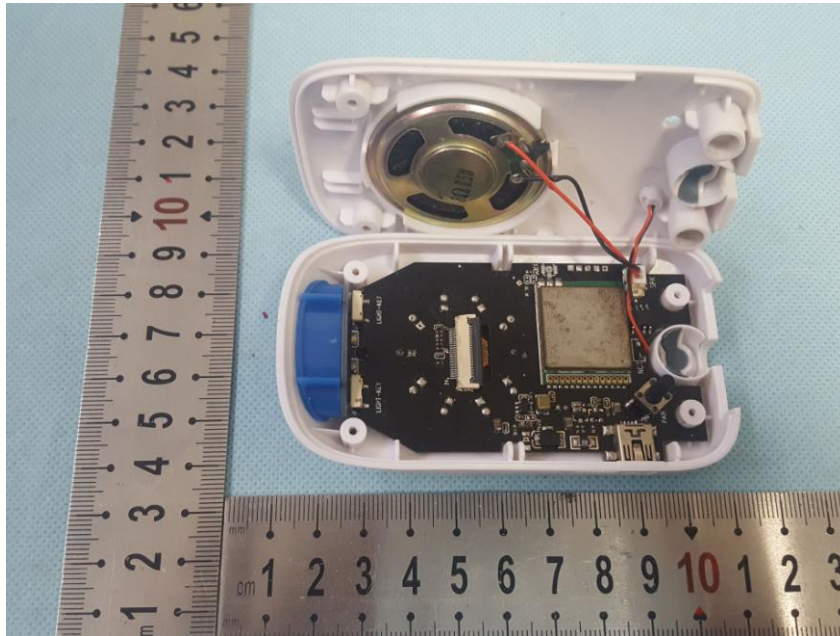
EUT Photo 5
