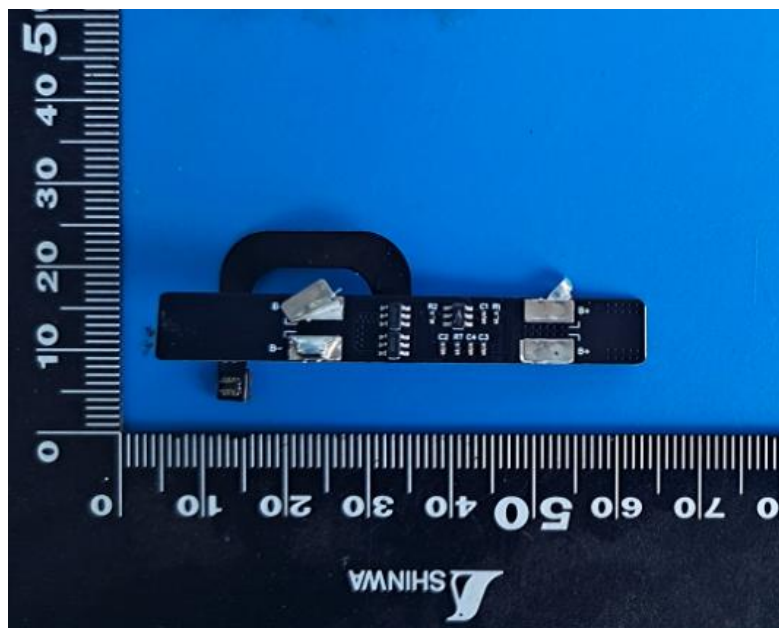
Fig. 5 – Front view of PCM 表5 – PCM 正面视图
