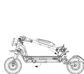
1.Aprire il gancio e sostenere la staffa di stazionamento.
