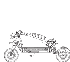
1. Ouvrez le crochet et soutenez le béquille.
