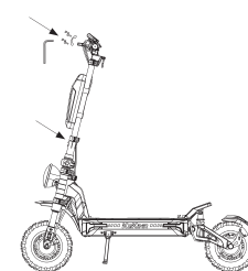
3.Serrare il blocco di bloccaggio del manubrio con le viti, installare il manubrio e la borsa appesa e accendere la macchina per verificare.
